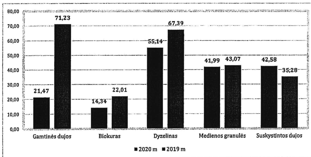
4 pav. Kuro sąnaudų palyginimas 1 MWh šilumos pagaminti, Eur
